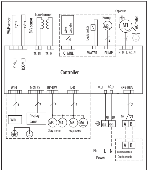
SACF48,60D5-A
