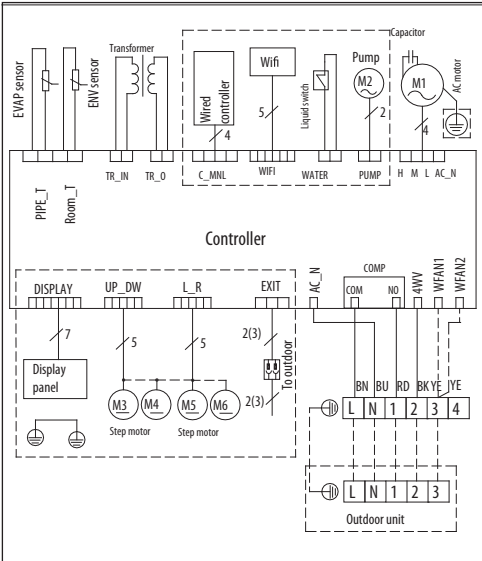
SACF24,36D5-A
