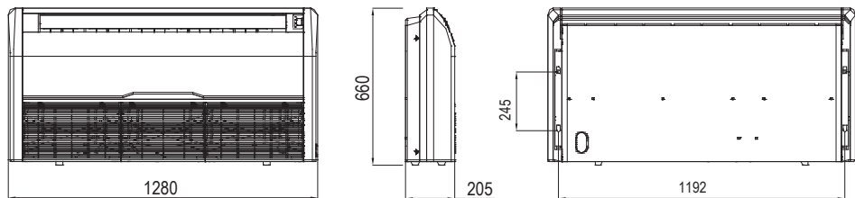
SACF24,36D5-A
