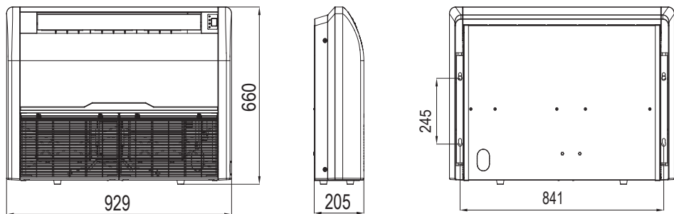
SACF18D5-A
